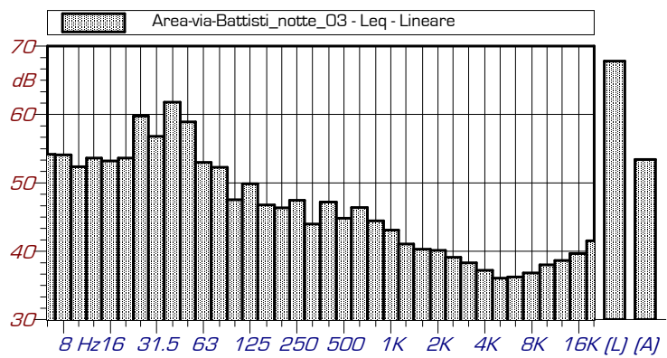
Area-via-Battisti_notte_03 - 1/3 Leq Spectrum + SLM - Lineare
