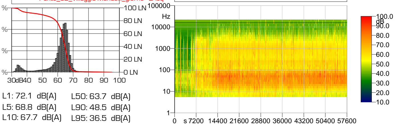
Punto_02_Villaggio-Mandelli_giorno - 1/3 Leq Spectrum + SLM - Lineare
