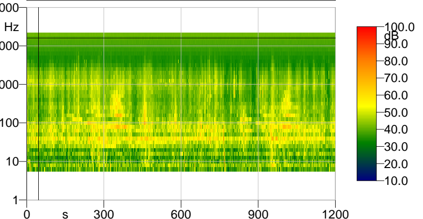
Area-via-Battisti_notte_01 - 1/3 Leq Spectrum + SLM - Lineare
