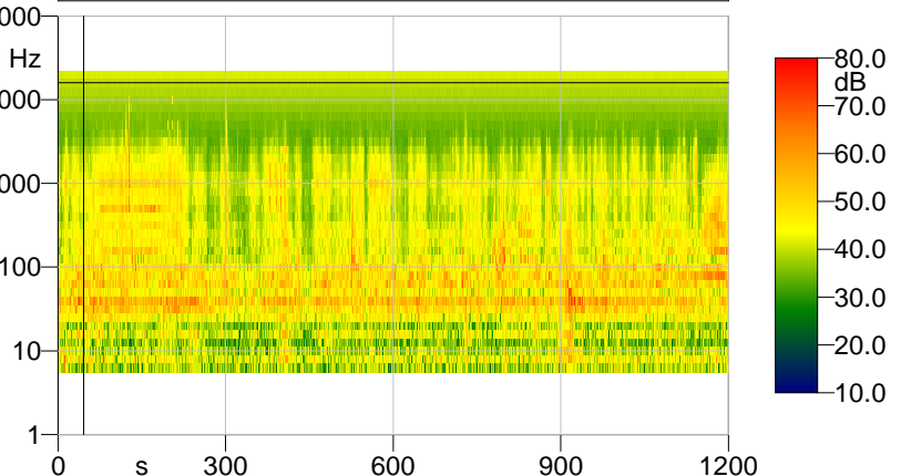
Area-via-Battisti_notte_02 - 1/3 Leq Spectrum + SLM - Lineare
