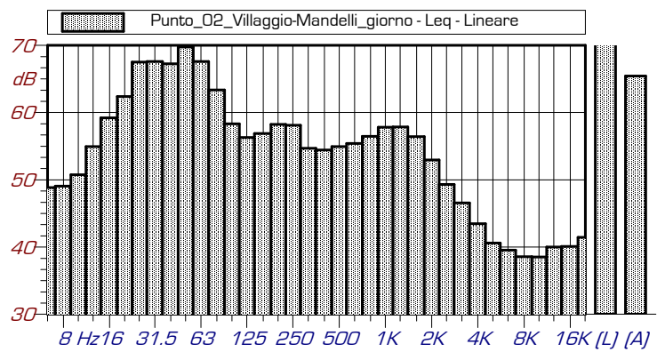
Punto_02_Villaggio-Mandelli_giorno - 1/3 Leq Spectrum + SLM - Lineare
