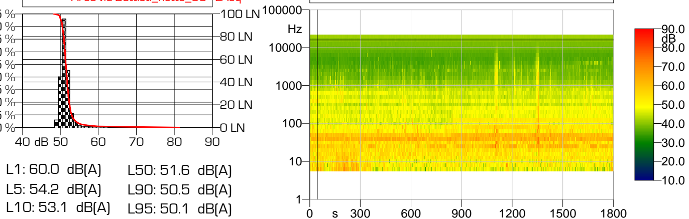
Area-via-Battisti_notte_03 - 1/3 Leq Spectrum + SLM - Lineare
