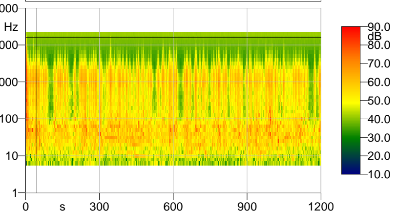
Area-via-Battisti_giorno_02 - 1/3 Leq Spectrum + SLM - Lineare
