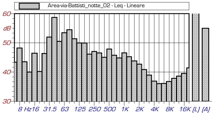
Area-via-Battisti_notte_02 - 1/3 Leq Spectrum + SLM - Lineare
