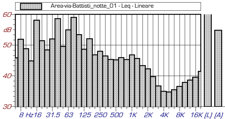
Area-via-Battisti_notte_01 - 1/3 Leq Spectrum + SLM - Lineare
