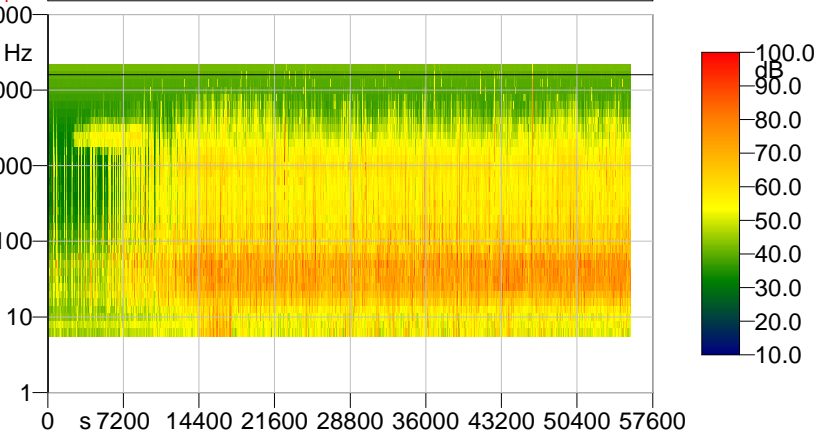
Punto_03_Villaggio-Mandelli_giorno - 1/3 Leq Spectrum + SLM - Lineare
