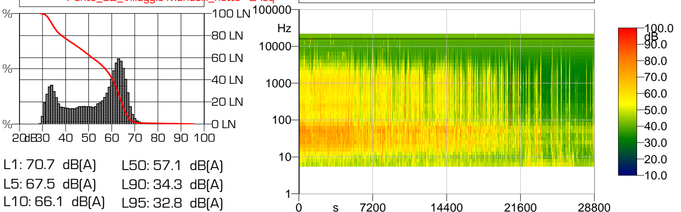
Punto_02_Villaggio-Mandelli_notte - 1/3 Leq Spectrum + SLM - Lineare
