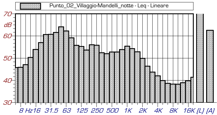
Punto_02_Villaggio-Mandelli_notte - 1/3 Leq Spectrum + SLM - Lineare
