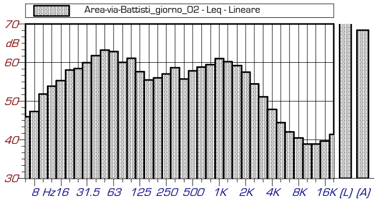
Area-via-Battisti_giorno_02 - 1/3 Leq Spectrum + SLM - Lineare
