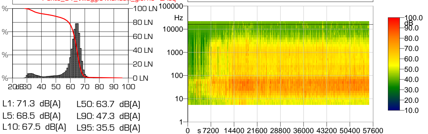
Punto_01_Villaggio-Mandelli_giorno - 1/3 Leq Spectrum + SLM - Lineare
