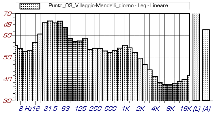
Punto_03_Villaggio-Mandelli_giorno - 1/3 Leq Spectrum + SLM - Lineare
