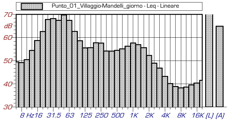
Punto_01_Villaggio-Mandelli_giorno - 1/3 Leq Spectrum + SLM - Lineare
