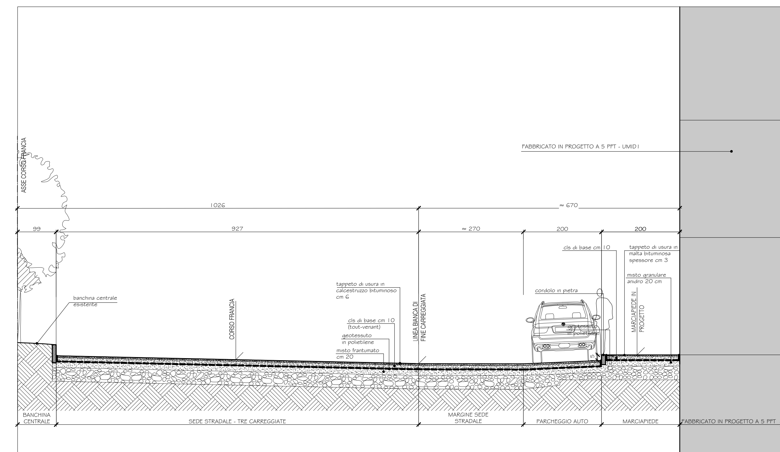
SEZIONE X-X IN PROGETTO DI VARIANTE - SCALA 1:50
