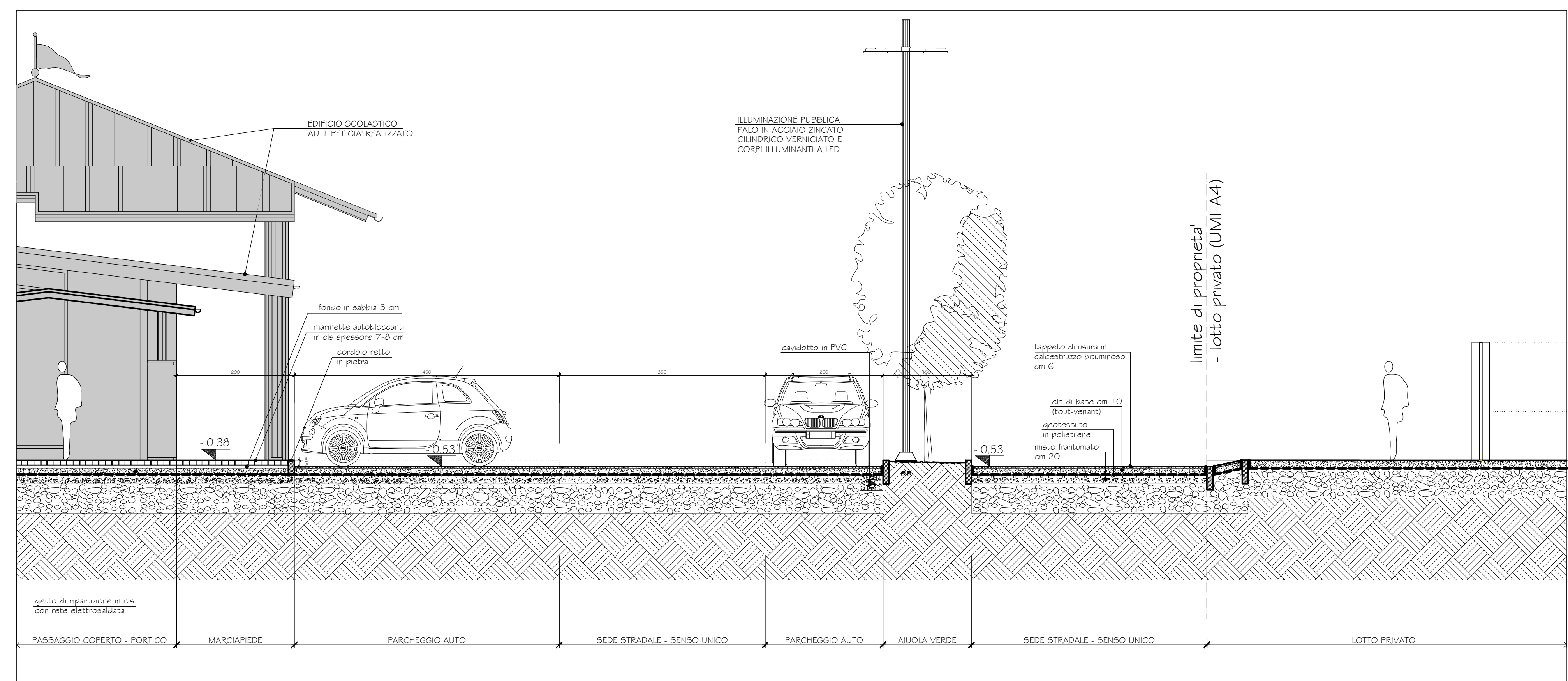
SEZIONE B-B IN PROGETTO DI VARIANTE - SCALA 1:50
