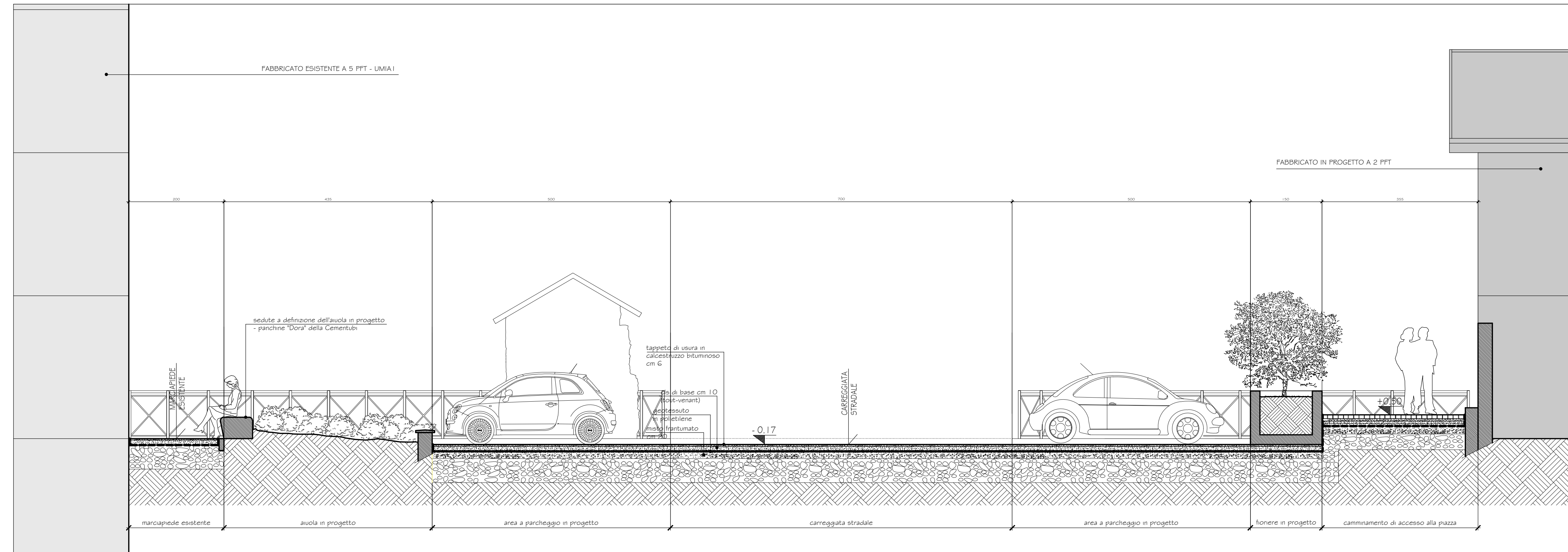
SEZIONE A-A IN PROGETTO DI VARIANTE (SUB-AMBITO A) - SCALA 1:50
