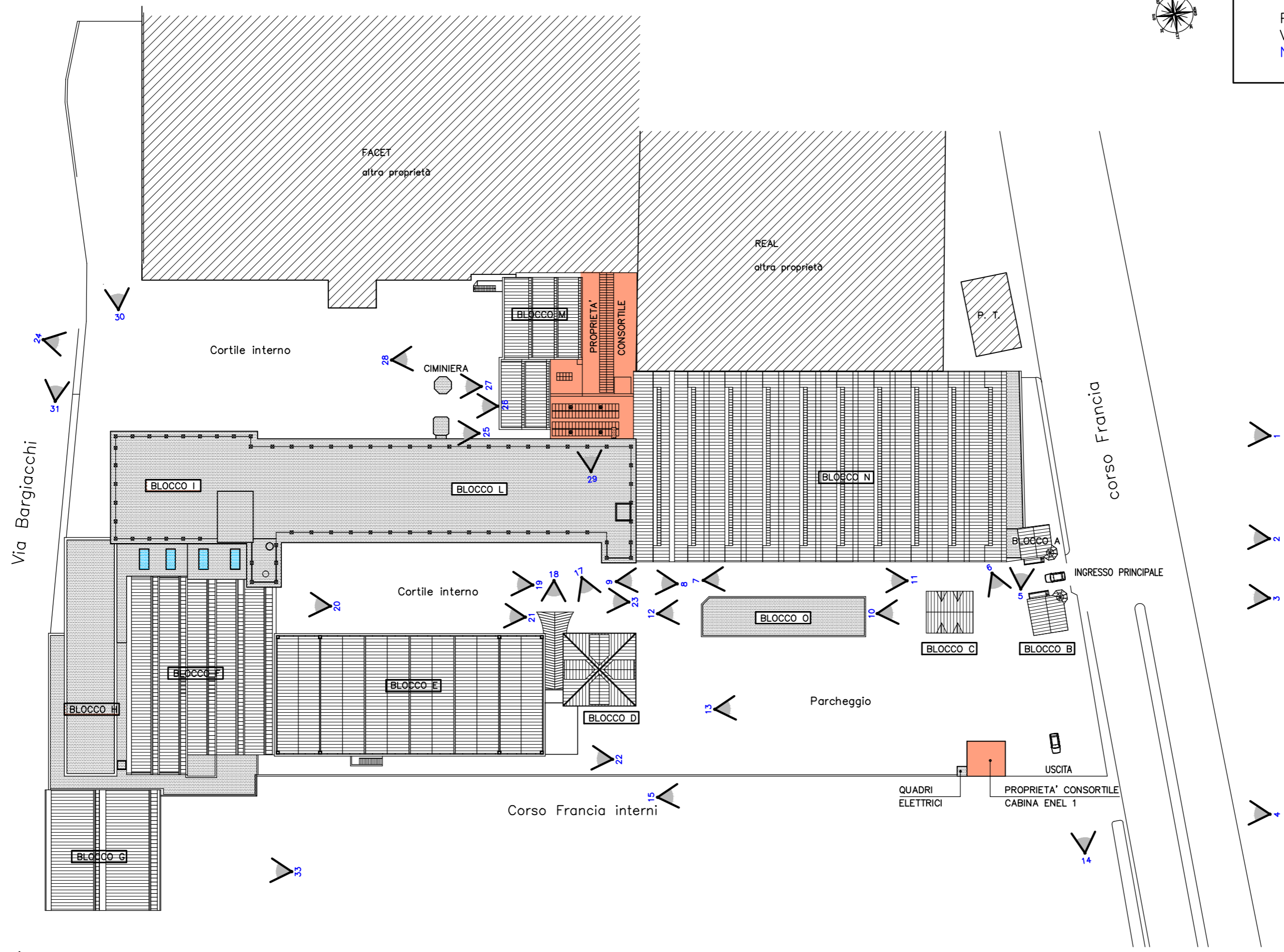
PLANIMETRIA GENERALE STATO DI FATTO VISUALIZZAZIONE RIFERIMENTI FOTOGRAFIE
